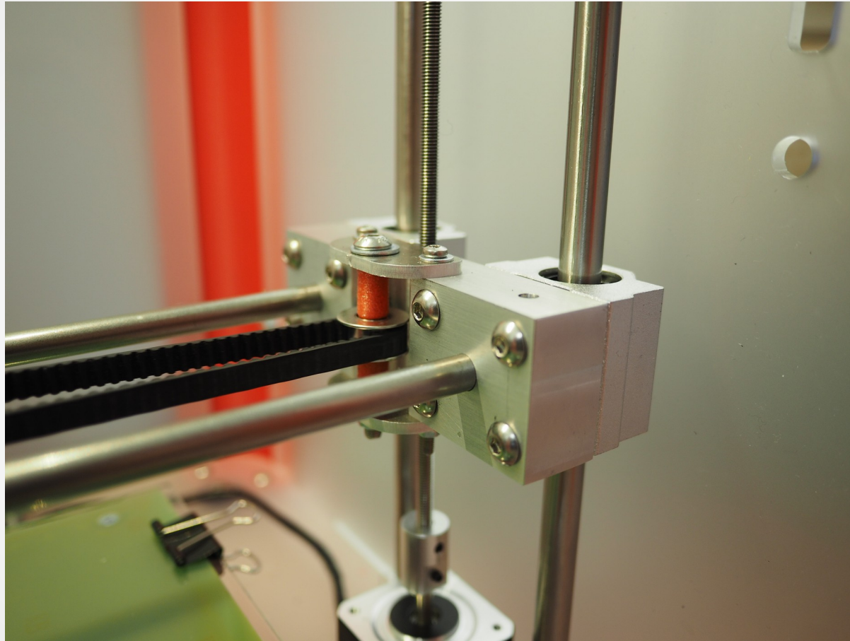
Détail mécanique de la Tobeca 3
