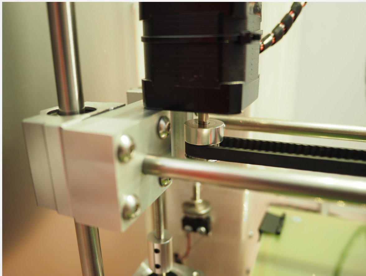
Détail mécanique de la Tobeca 3
