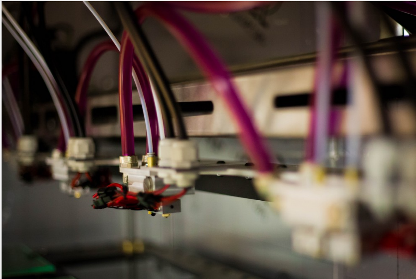
Vue de détail des têtes de l'imprimante multi plateaux Tobeca 5X2
