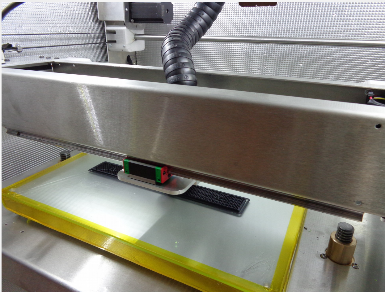
Détail du chariot de la Tobeca 336, ombilical, guidages et plateau rectifié
